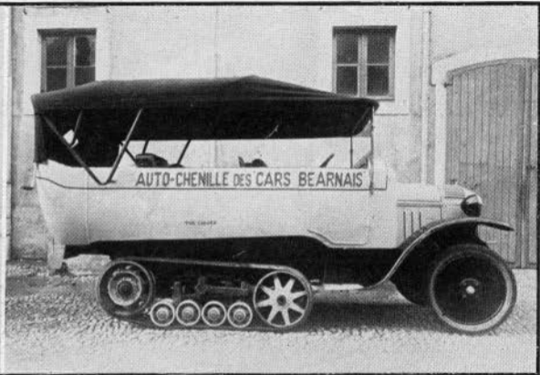
Car de montagne carrossé sur châssis Citroën muni du propulseur Kégresse-Hinstin.
