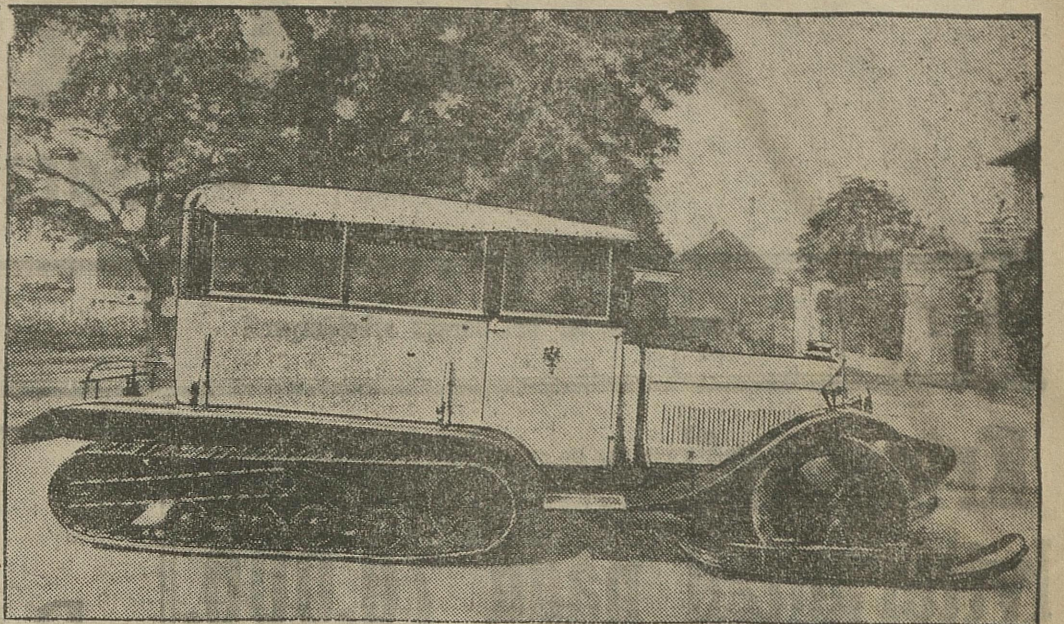
Vi bringer her et bilde av en ny slags beltebil som det østerrikske postvesenet har innført. Den har allerede vist sig meget effektiv ved postbefordringen på de isete fjellveier i Tirol.
