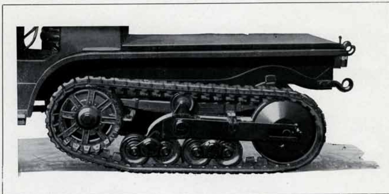
PROPULSEUR KÉGRESSE-HINSTIN ENTRAÎNEMENT SILENCIEUX - BANDAGES MÉTALLO-CAOUTCHOUC
