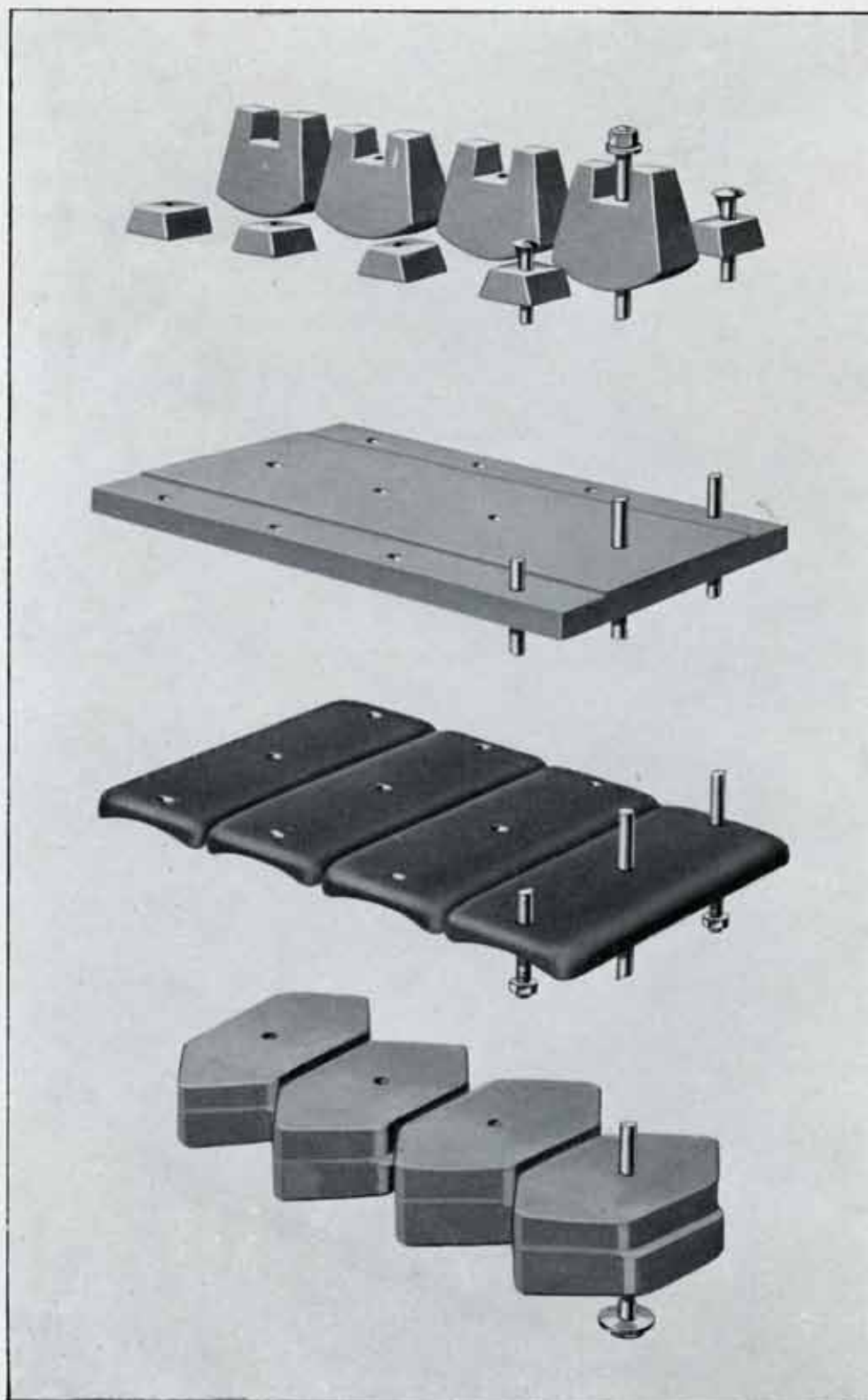
DÉTAIL DU BANDAGE MÉTALLO-CAOUTCHOUC
