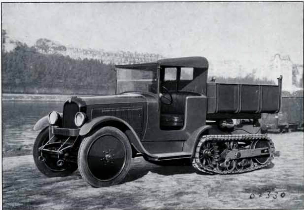
BENNE BASCULANTE POUR L'ENLÈVEMENT DES ORDURES MÉNAGÈRES
