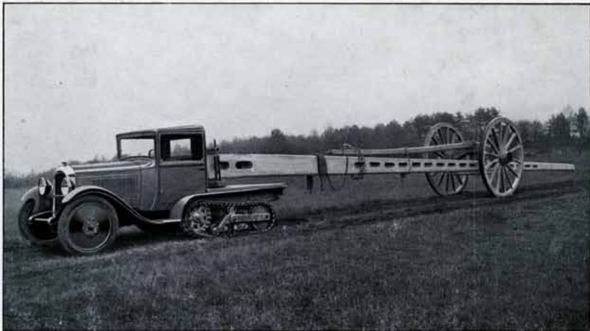
AUTOCHENILLE CITROËN REMORQUANT UN PYLONE D'ÉLECTRIFICATION A TRAVERS TERRES
